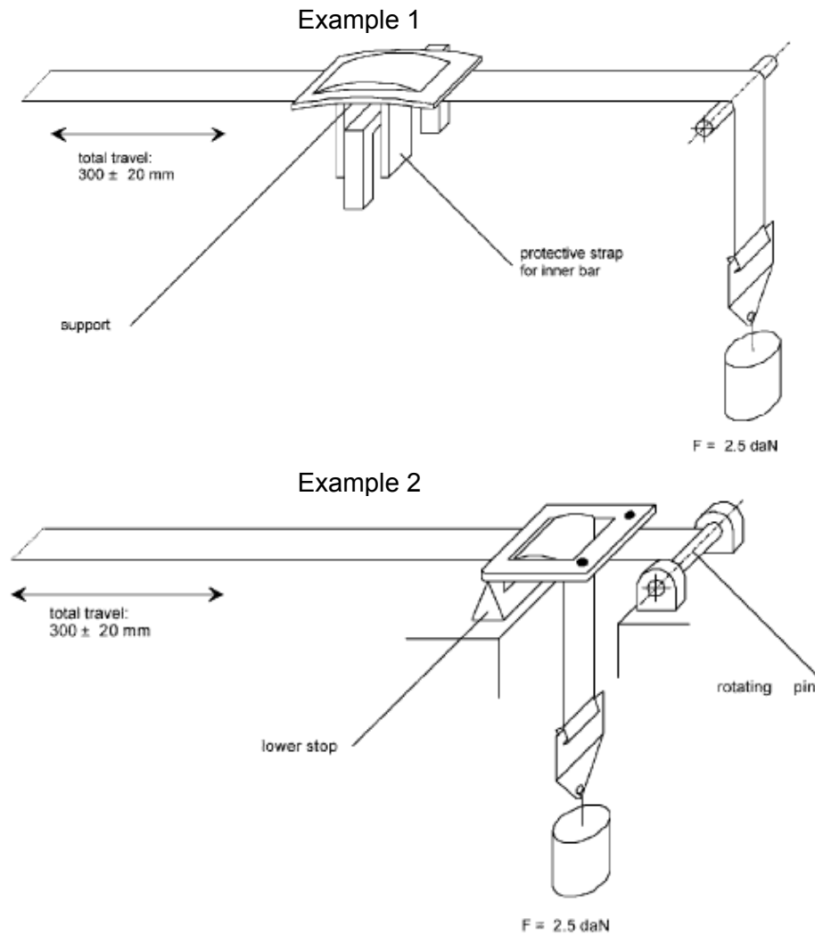
Fig 3. Type-1 abrasion
