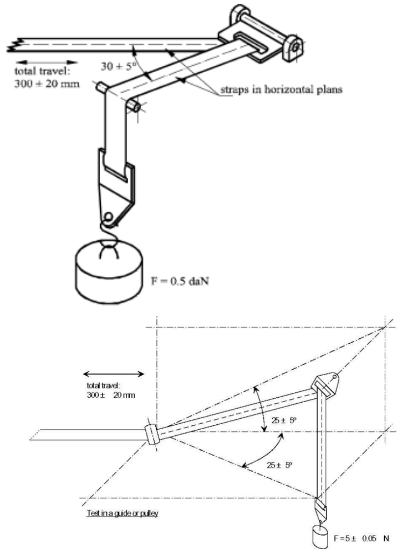
Fig 4. Type-2 abrasion
