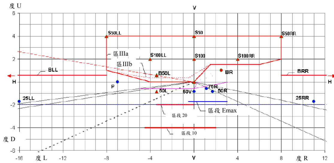
圖1 近光光束光度量測點
