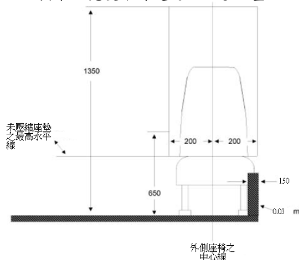
圖一：下方乘客空間之允許侵入範圍
