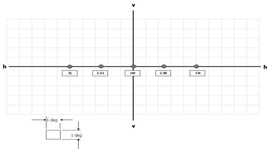
圖二：近光燈量測點位置
