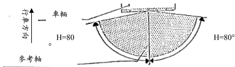
圖三：L類車輛單燈式尾燈水平照射角度
