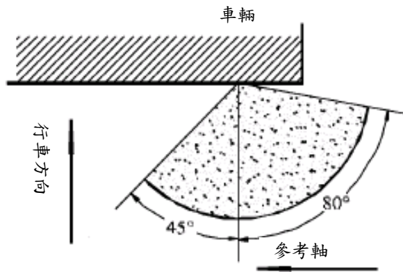
圖二：M、N、O類車輛尾燈及L類車輛成對尾燈水平照射角度
