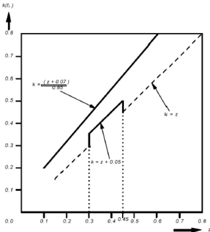
圖一 A 6.6.1.2.1所述N1類車輛
