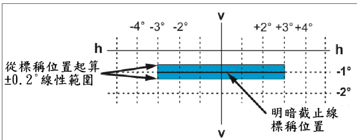
圖五：明暗截止線形狀和位置
