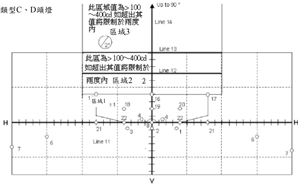
圖四：對稱光型頭燈配光螢幕
