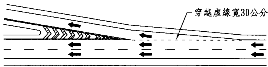
單車道直接式出口
