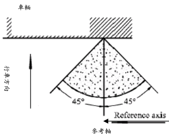
圖二 煞車燈參考軸
