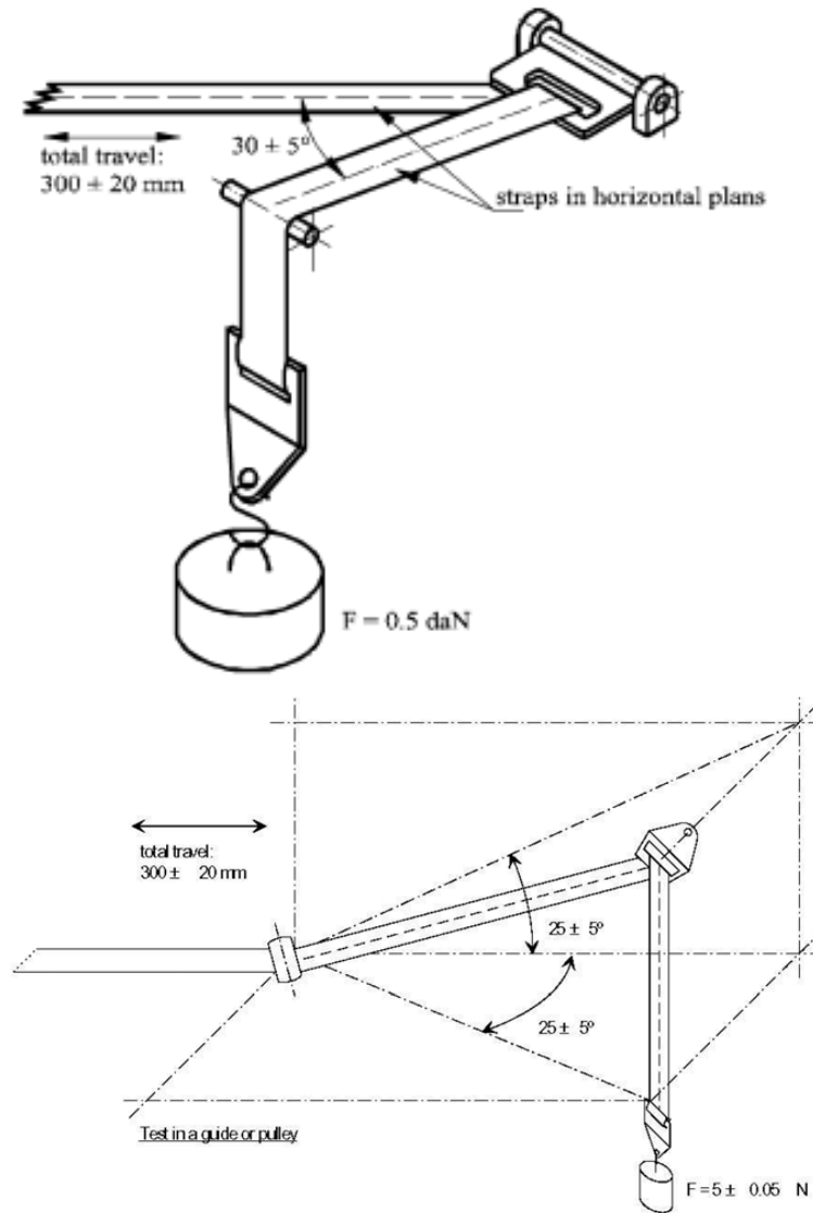
Fig 4. Type-2 abrasion
